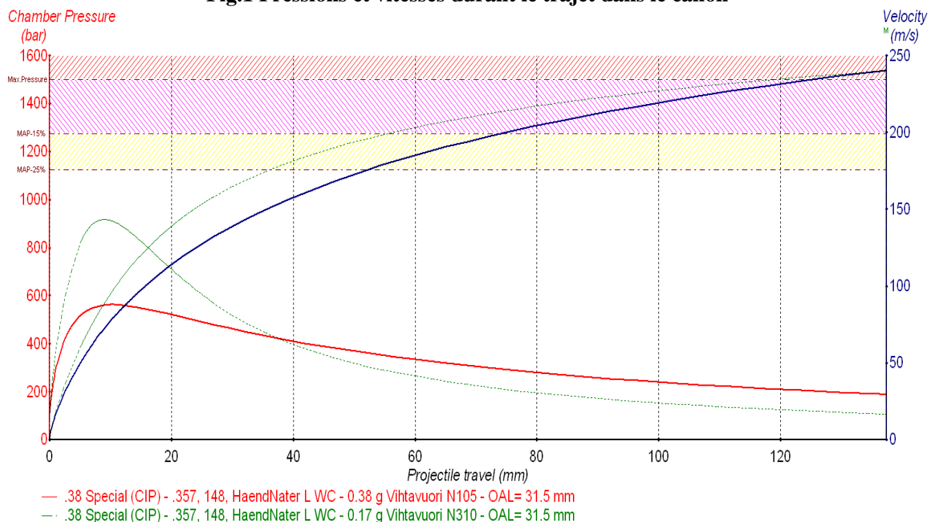
Fig.1 Pressions et vitesses durant le trajet dans le canon
