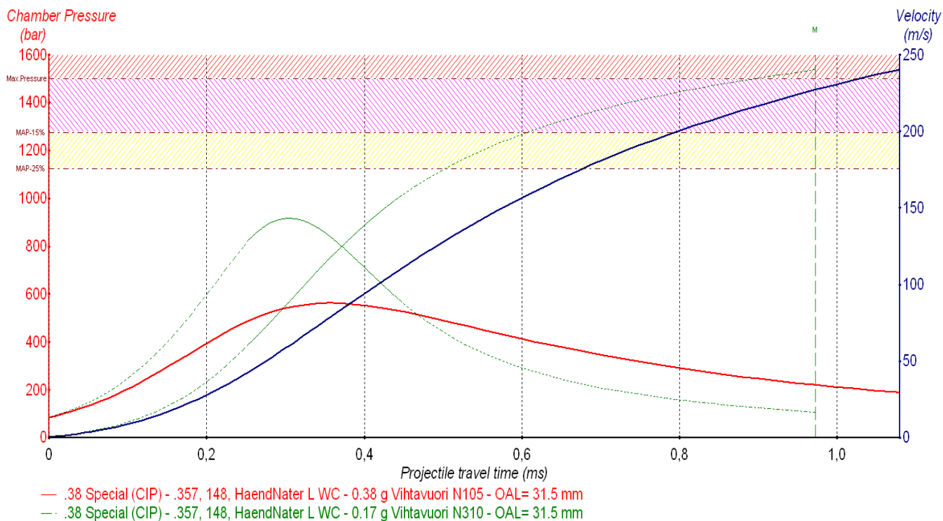
Fig.3 Pressions et vitesses en fonction du temps de trajet
