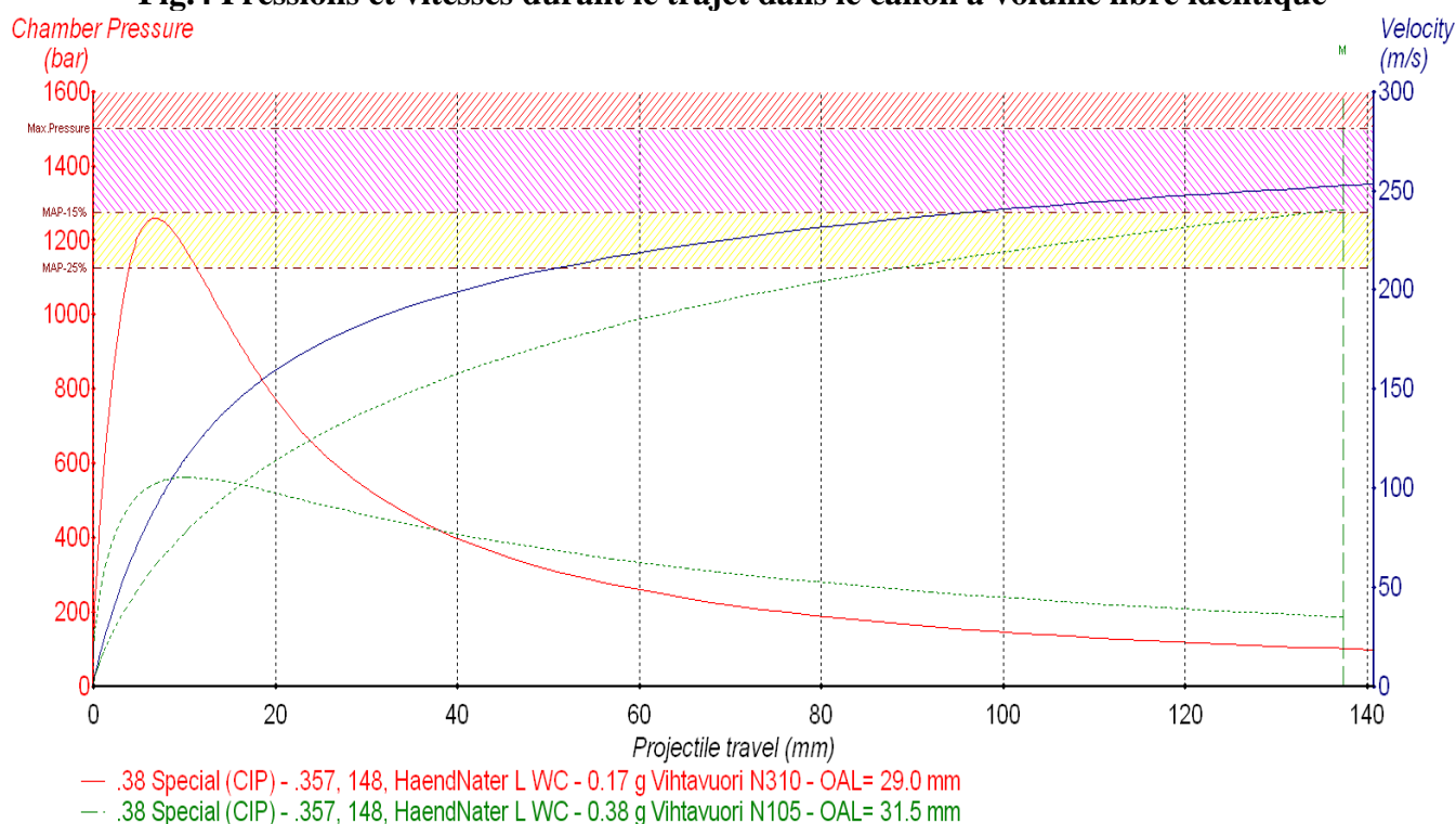
Fig.4 Pressions et vitesses durant le trajet dans le canon à volume libre identique
