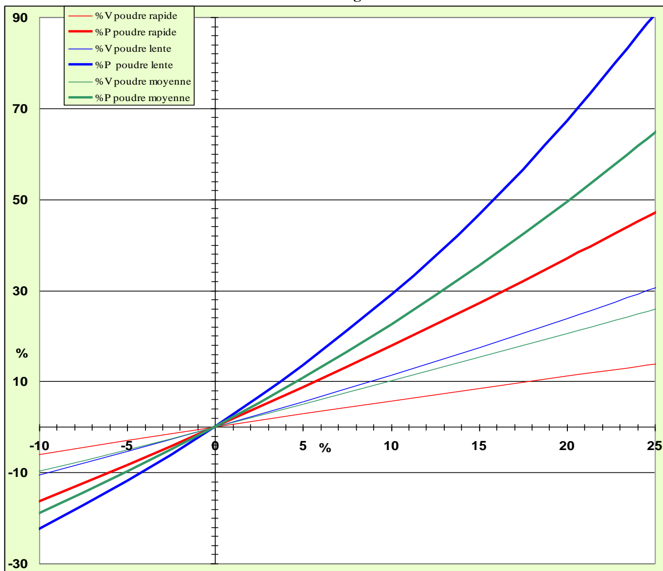
Fig.5 Pourcentage de Variation de vitesse et de pression en fonction du pourcentage de la variation de charge
