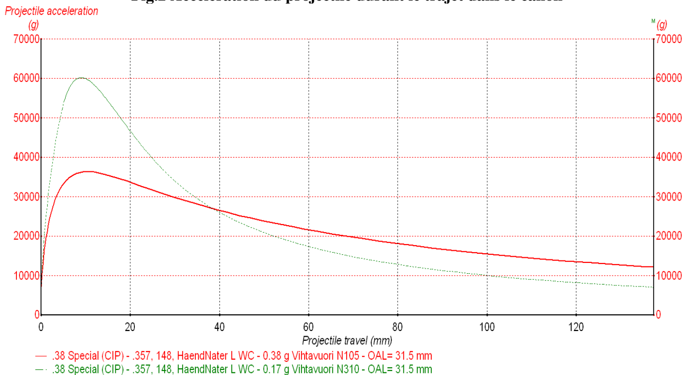
Fig.2 Accélération du projectile durant le trajet dans le canon
